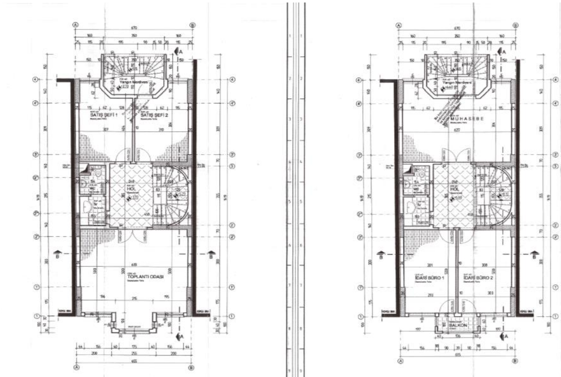
Birinci Kat ve İkinci Kat Planı:
