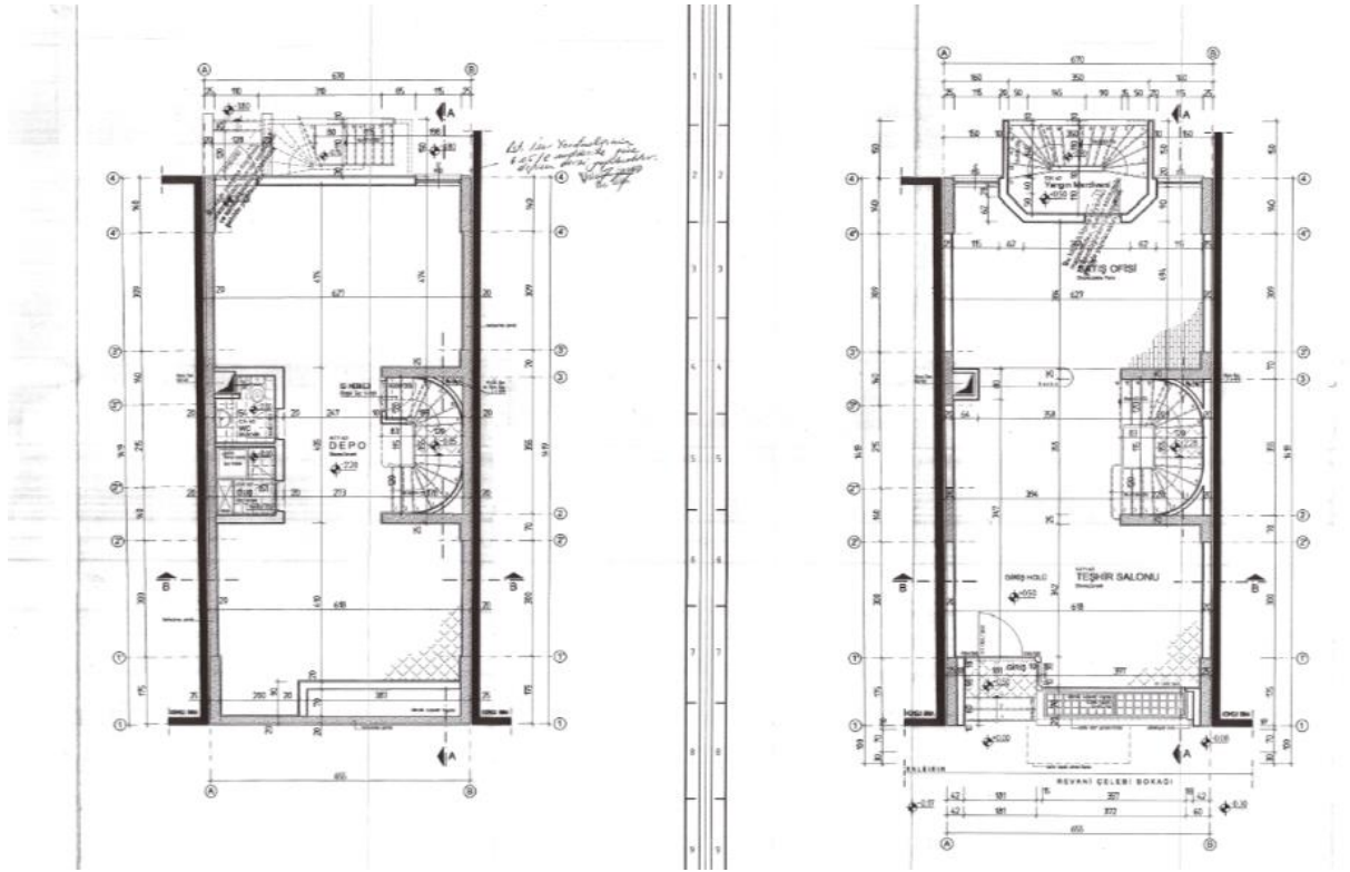
Birinci Kat ve İkinci Kat Planı:
